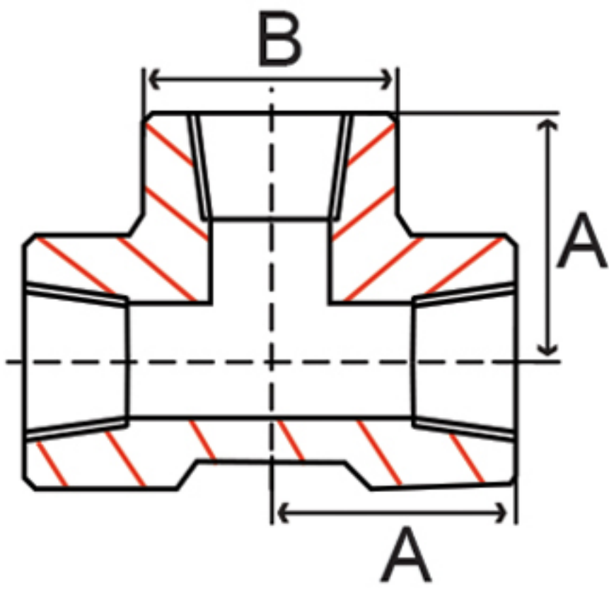
Fig. 42T 3 – Tee
